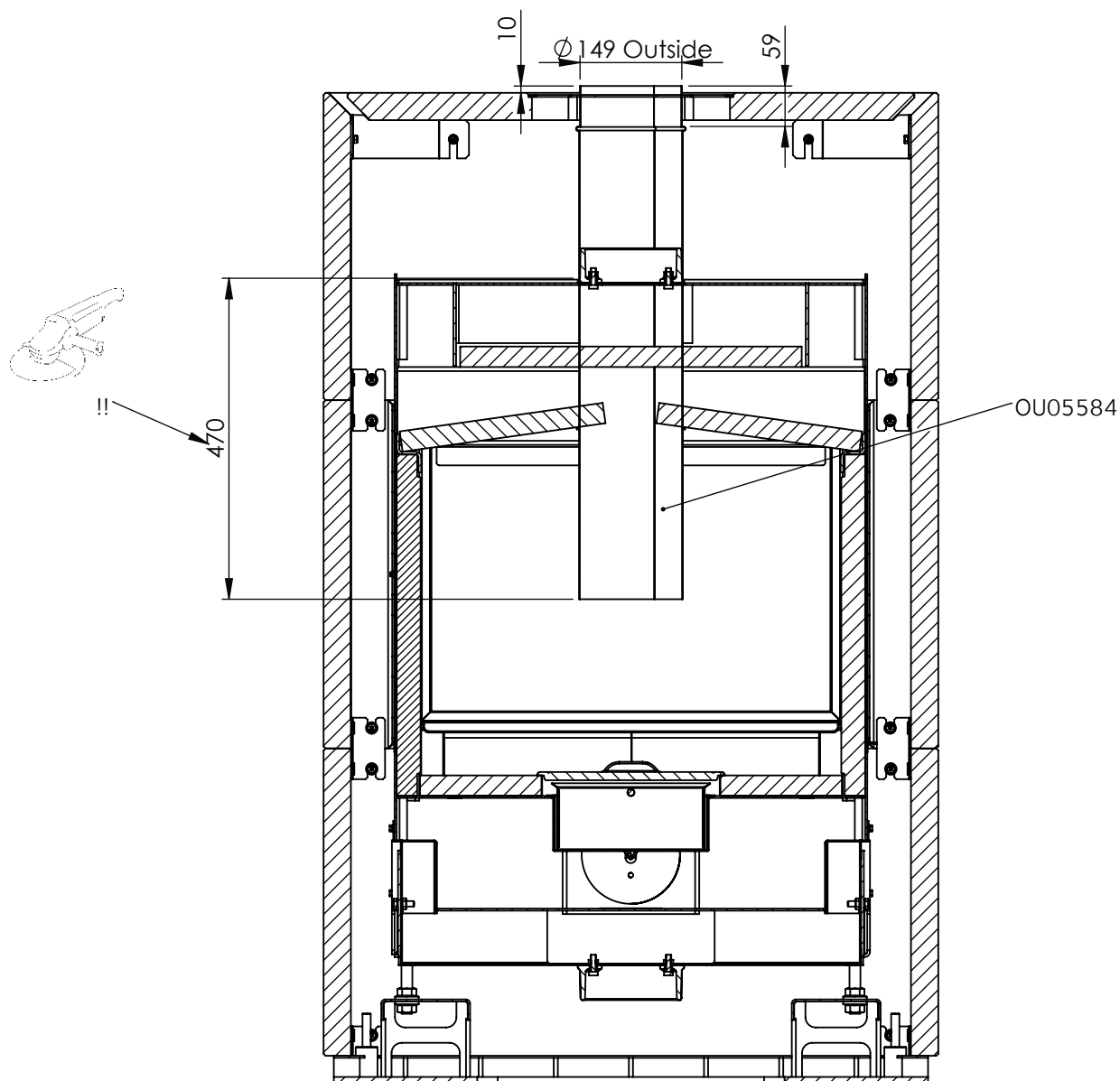
SECTION T-T SCALE 1 : 10
