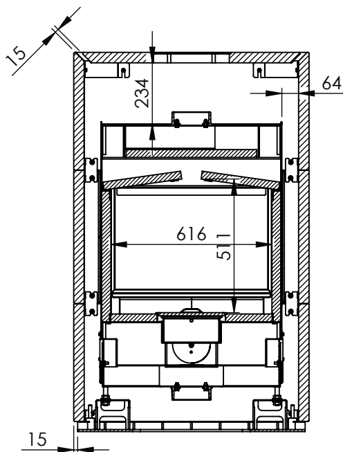
SECTION I-I SCALE 1 : 20
