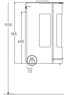
WESTFIRE.UNIQ.36 WESTFIRE.UNIQ.37 VEGGMONTERT / VEKT: 85 KG
