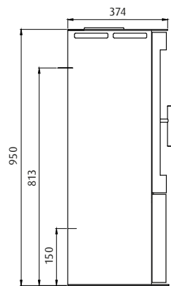
WESTFIRE.UNIQ.46 VEKT: 90 KG
