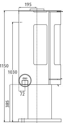
WESTFIRE.UNIQ.36 WESTFIRE.UNIQ.37 MED SOKKEL 1 / VEKT: 95 KG
