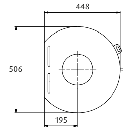
WESTFIRE.UNIQ.46 VEKT: 90 KG
