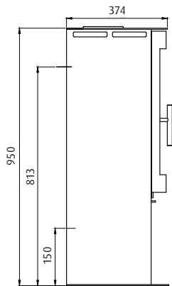
WESTFIRE.UNIQ.45 VEKT: 90 KG
