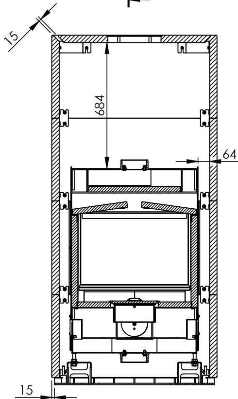
SECTION I-I SCALE 1 : 20
