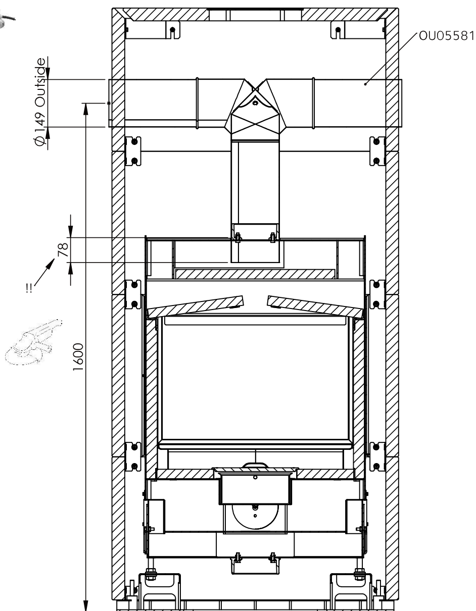
SECTION V-V SCALE 1 : 12
