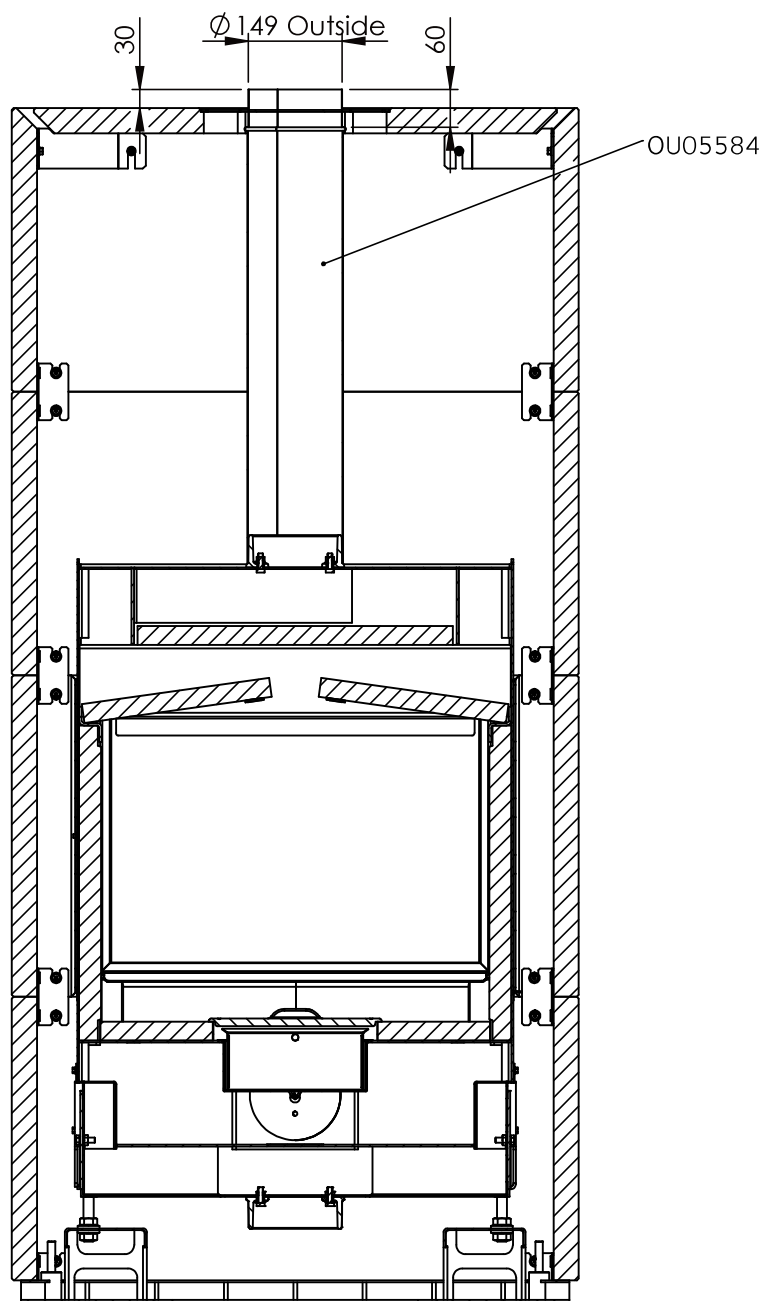
SECTION T-T SCALE 1 : 12
