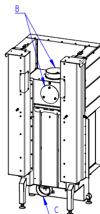
C. Primærluftinntak
