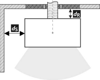
Hinterer Rauchrohranschluss
