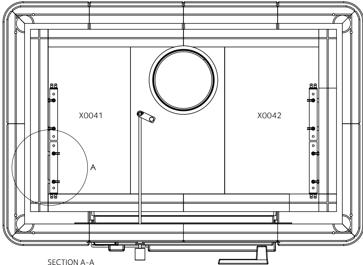
SECTION A-A SCALE 1 : 6
